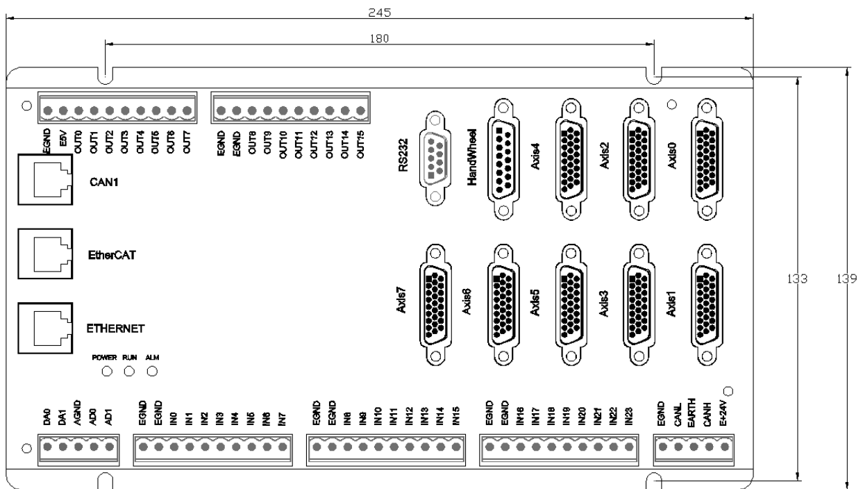
单位: mm 安装孔直径 4.5mm 厚度 52mm
