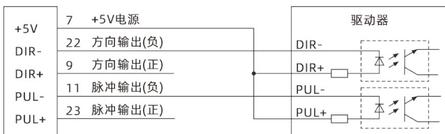
PUL/DIR 单端接线示意图:
