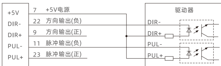
PUL/DIR 共阳极接线示意图:
