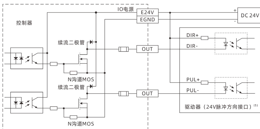
注[1]: 针对于5V的脉冲方向接口, PUL+和DIR+请连接到E5V接口。
