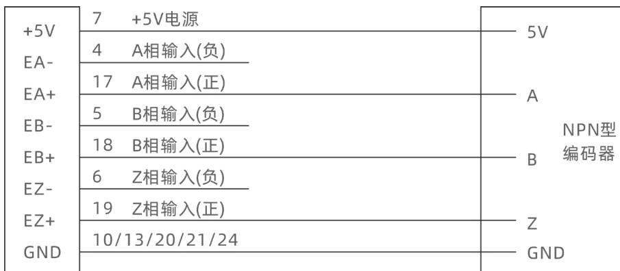
EA/EB/EZ 单端接线示意图:
